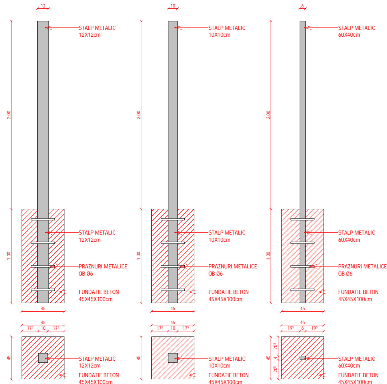
■ DETALIU FUNDATIE
